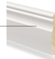
PÕRANDALIIST Värvitud männipuidust põrandaliist 18x95mm Värvitud uksega sama tooni- RAL9010. Profiil nr.18, www.siivik.ee
